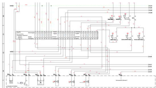
Projeto elétrico
